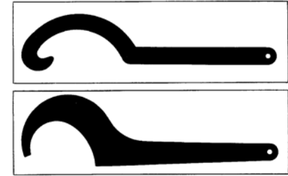
第 1－1 図 キャップスバナ
